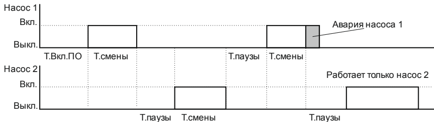
Рисунок 3.1 - Диаграмма переключения насосов
