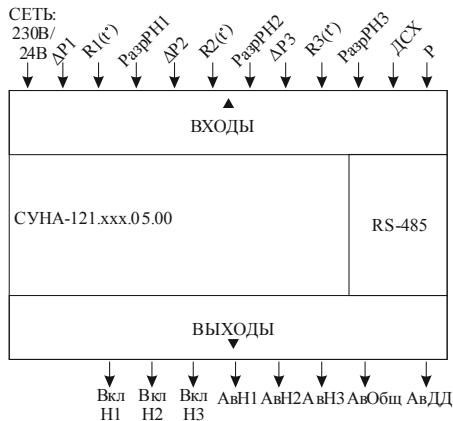
Рисунок 2.1 - Схема объекта управления
