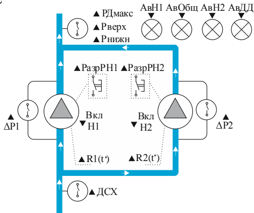
Рисунок 2.1 - Схема объекта управления
