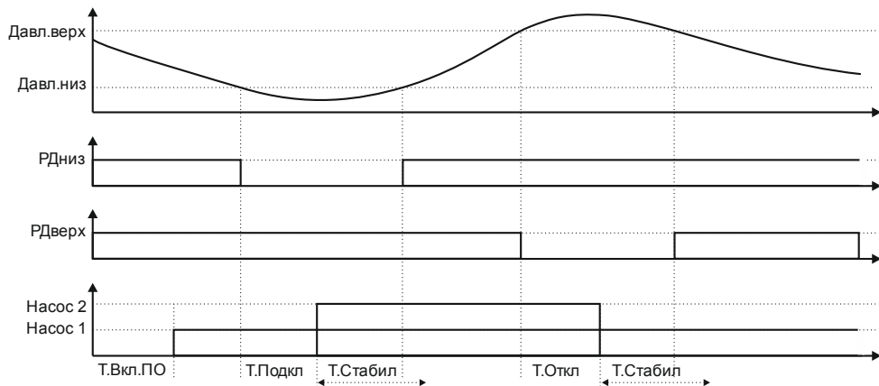
Рисунок 3.2 – Диаграмма работы насосов при поддержании давления
